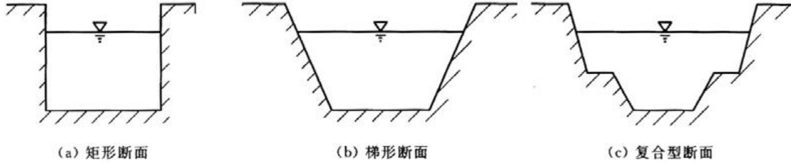
图1 滑坡地面排水沟断面形状示意图
