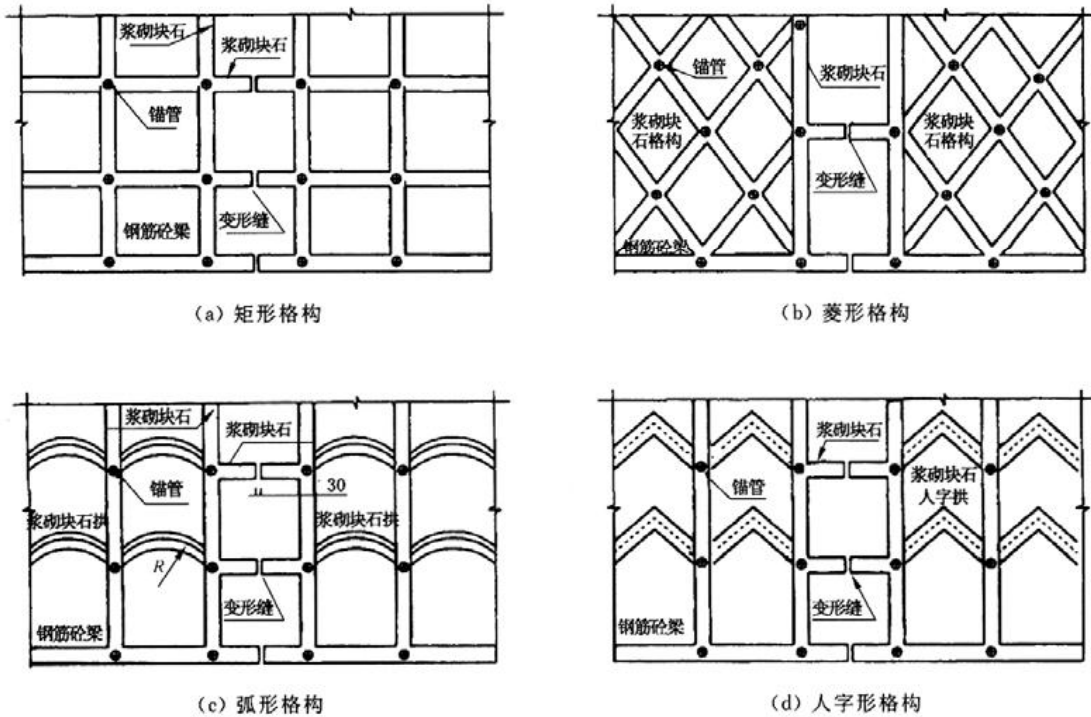
图 7 格构平面布置型式图
