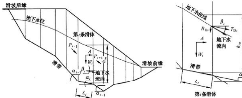
图 A.2 传递系数法(折线型滑动面)(堆积层滑坡计算模型之二)
